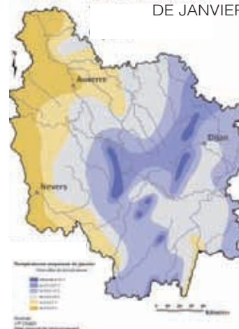
TEMPÉRATURES MOYENNES DE JANVIER
